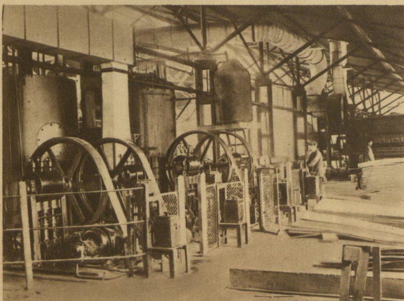
Гідраўлічныя помпы і акумулятары да іх (да 400 атмасфэр ціску) для фанэрных прэсаў
