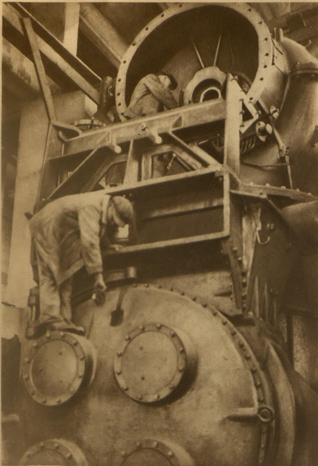
Устаноўка турбагенэратара на 10.000 квт.
