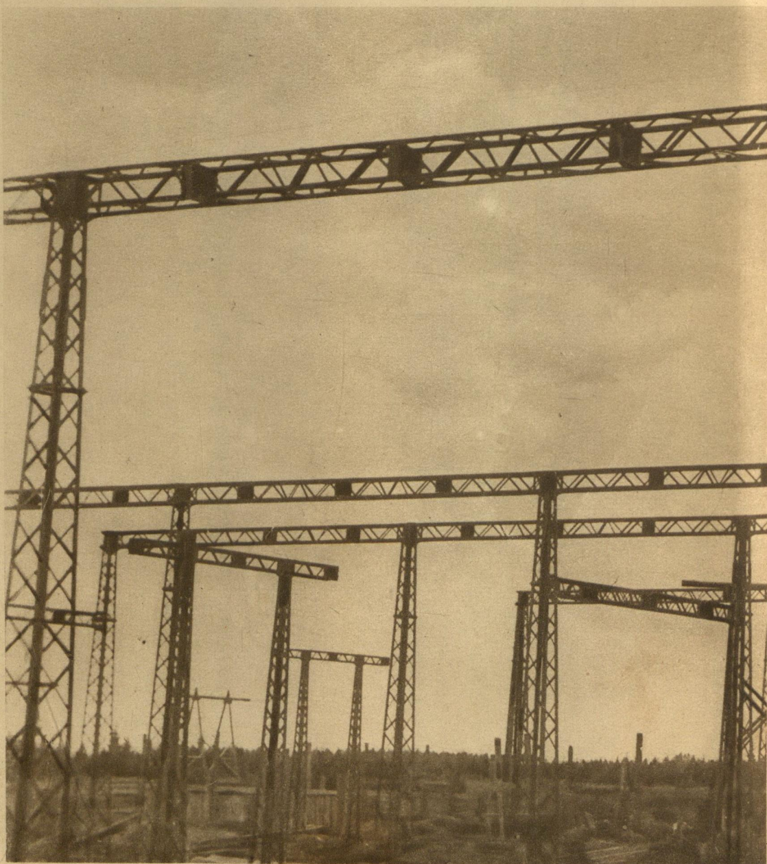
Адкрытая частка падвышальнай падстанцыі (на 110.000 вольт) Асінстану
