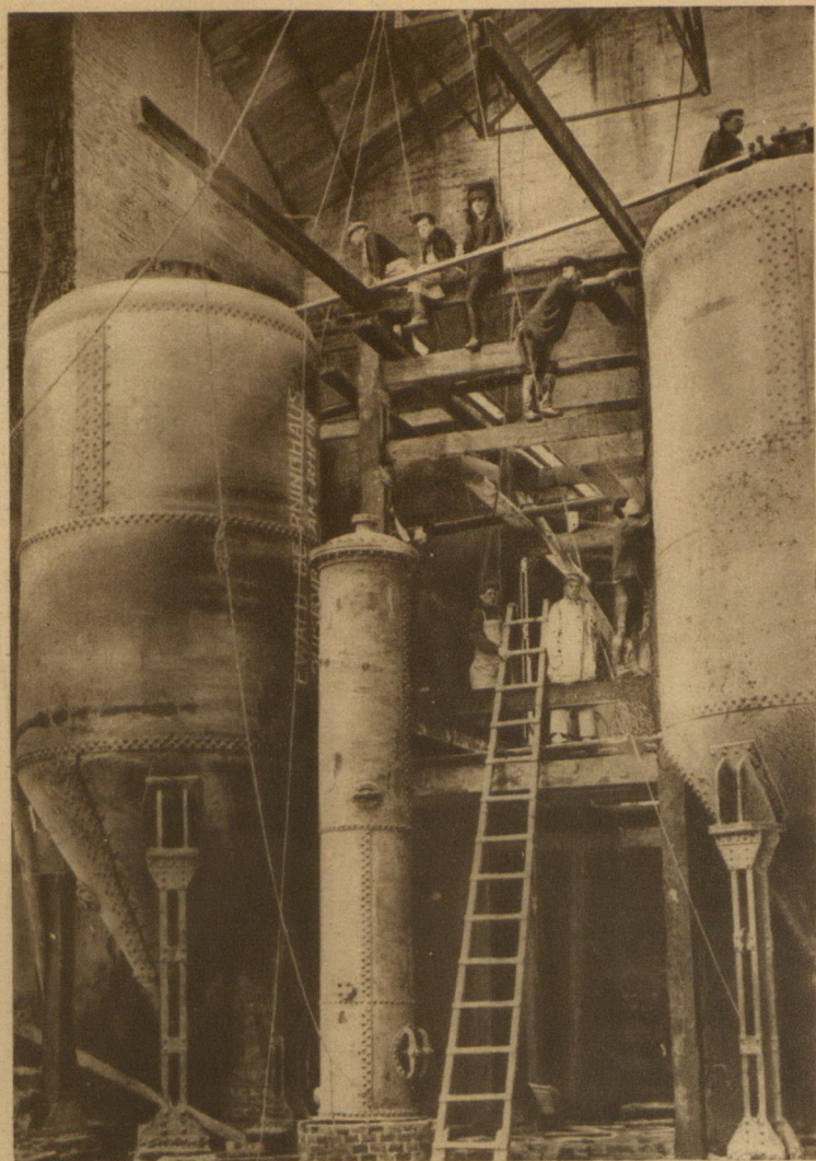
Устаноўка саломаварачных цыліндрычных катлоў на саламяна-цэлюлёзным заводзе
