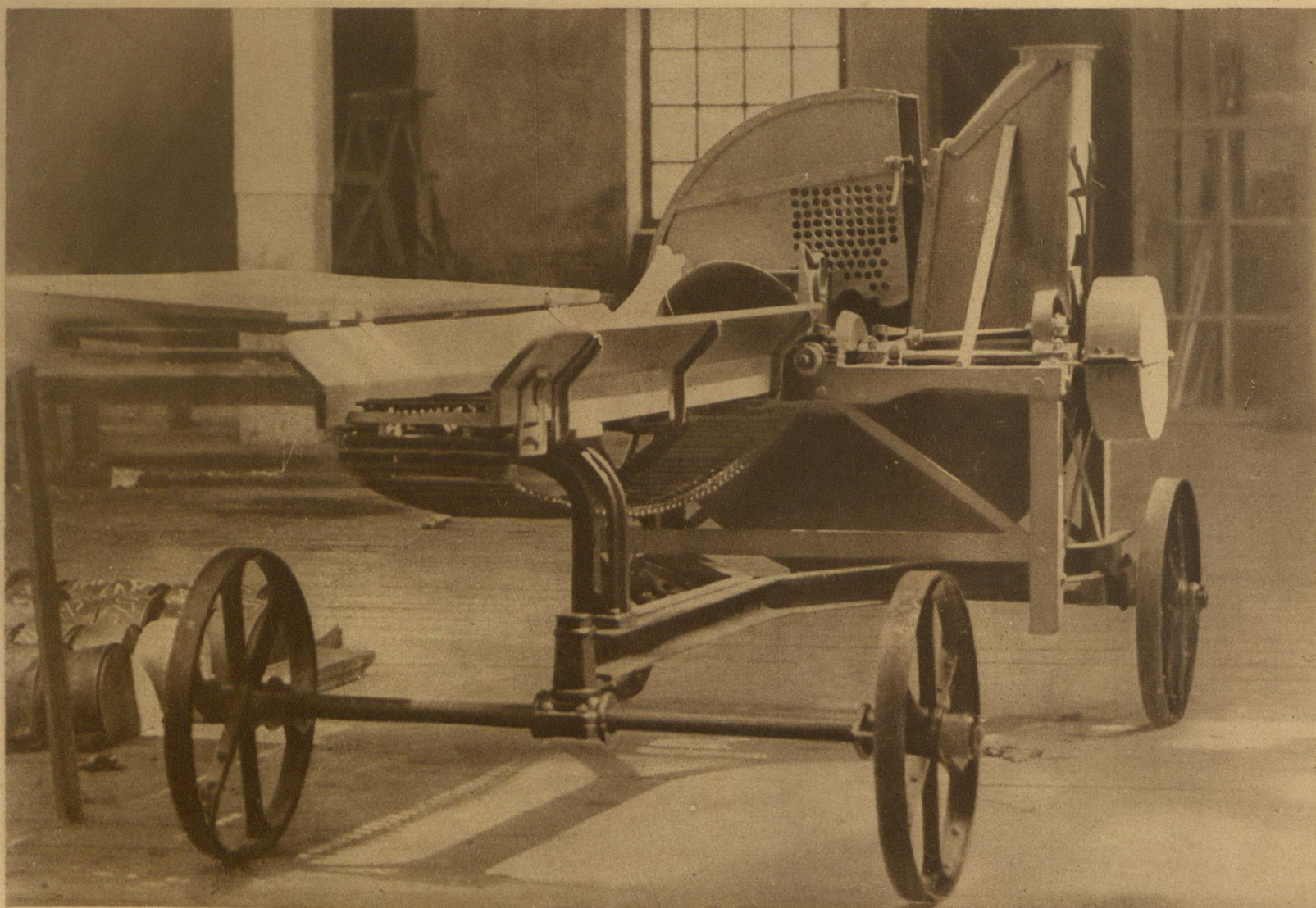
Сіласарэзка, выпушчаная заводам
