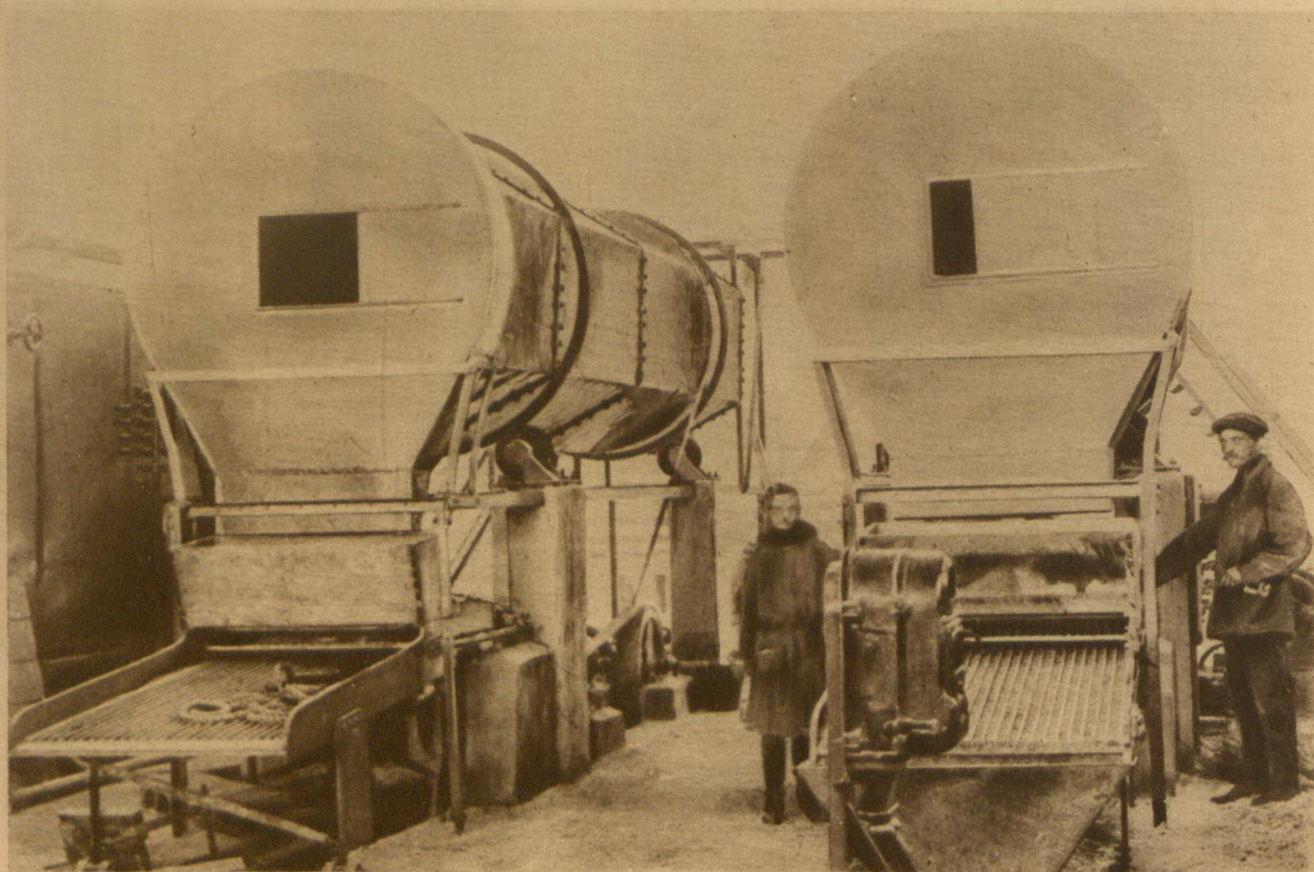
Барабаны для паліроўкі саломы
