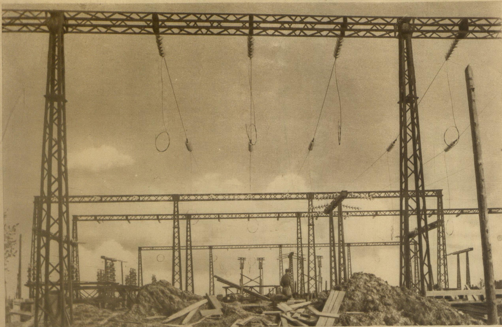
Частка Віцебскай паніжаючай падстанцыі на 110.000 вольт
