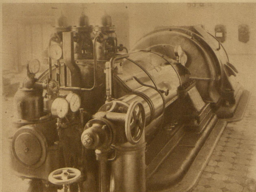
Турбагенэратар першай чаргі—1.250 квт.
